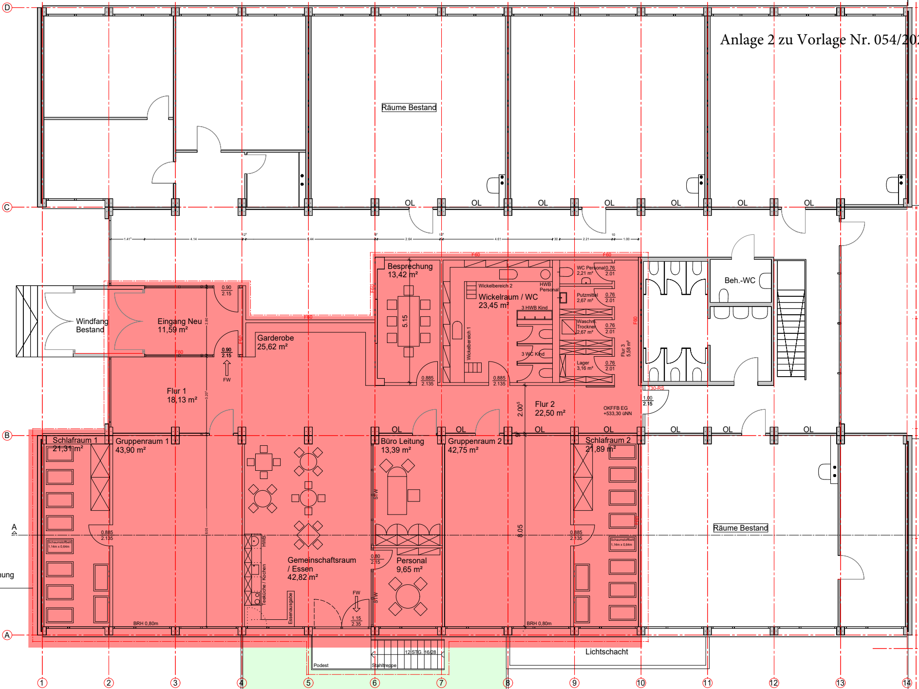
Übersicht Neuplanung EG: Umnutzung Teilfläche in Halbtageskinderkrippe
